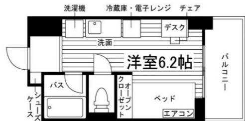
Fタイプ 1R (15.8㎡)
